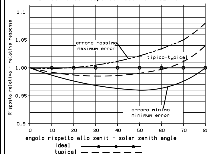
Risposta angolare (coseno + azimut) Directional response (cosine + azimuth)
