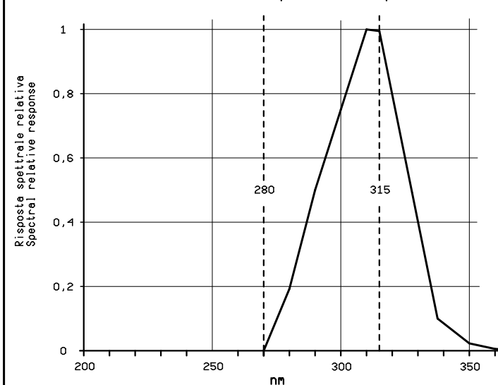
Risposta spettrale relativa Relative spectral response
